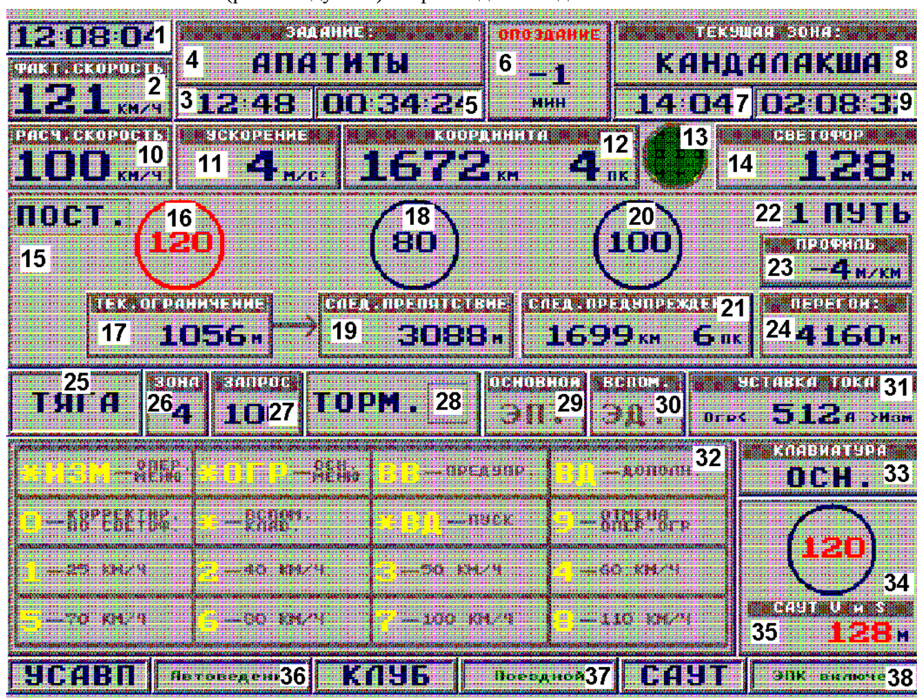
Рисунок 10 – Основной экран системы УСАПВ-ЭП1 для электровозов ЭП1 и ЭП1М
